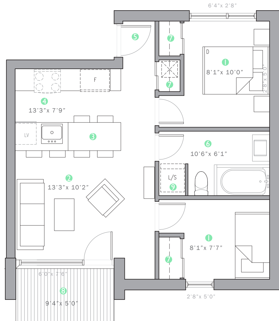
NIVEAU 2 (OPTION 1) - 593 PI.CA
