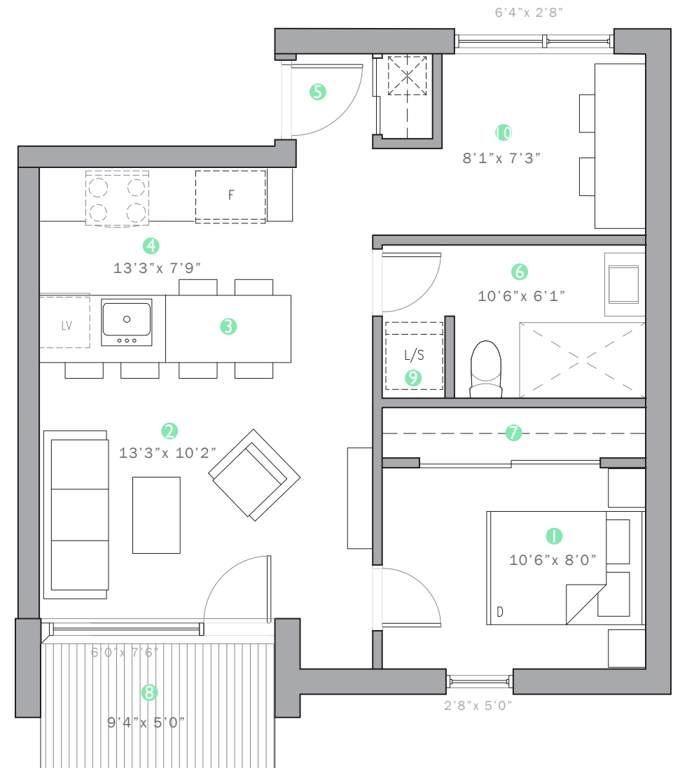
NIVEAU 2 (OPTION 2) - 593 PI.CA
